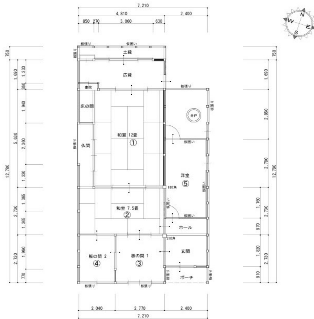
改修前平面図
