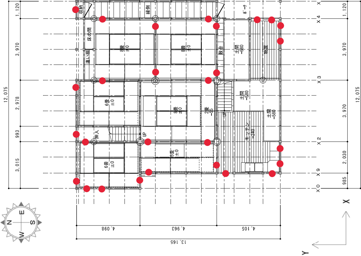
1 階制震ダンパー設置計画図
