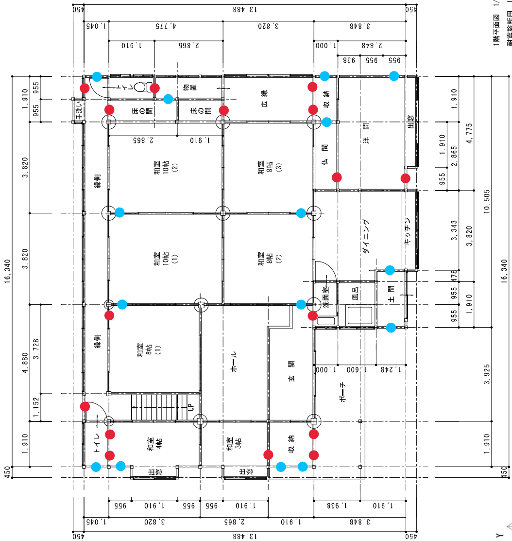
1階制震ダンパー設置計画図 S=1/100
